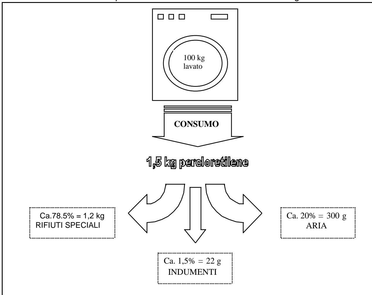
Schema 1: Bilancio di massa globale del percloretillene per il lavaggio di 100 kg di indumenti in un impianto della sesta generazione
